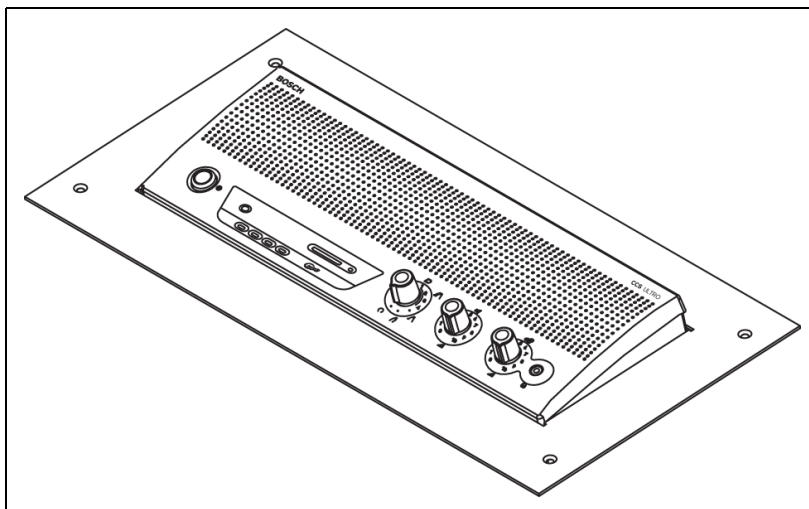
Рисунок 10.3 Установка в стол
