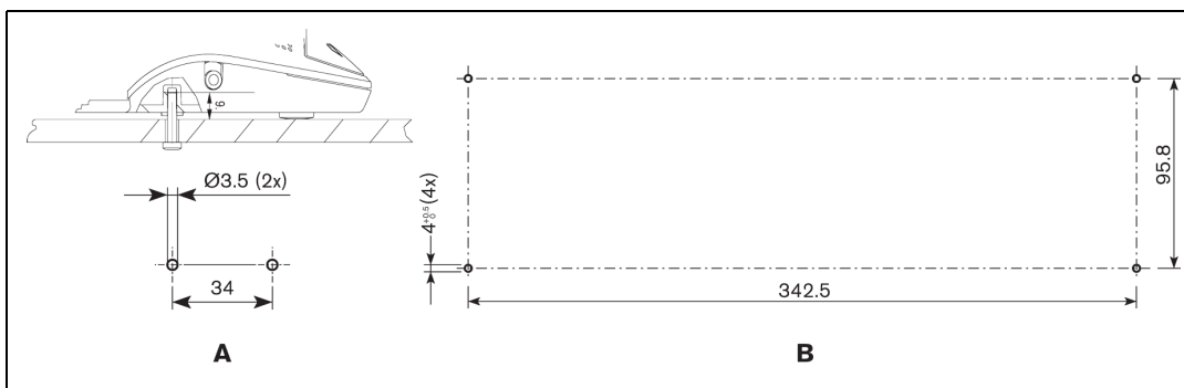
Рисунок 10.4 Установка на стол
